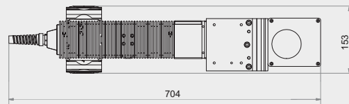
VL-GREEN
