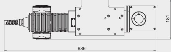
VL-UV
